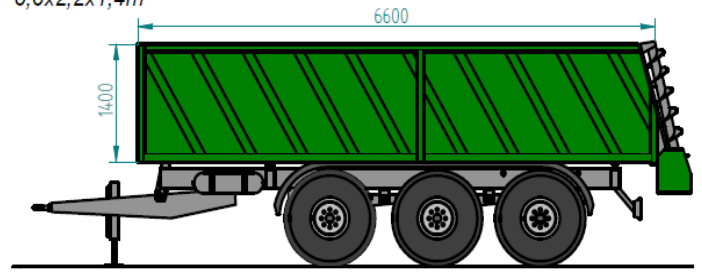
Agromax Plus T A180 TSZ 6,6x2,2x1,4m
