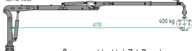
IGJ HD 3063
