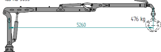
IGJ HD 3063
