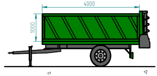
Agro 65 TSZ 4,0x1,8x1,0m
