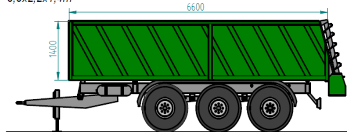
Agromax Plus T A180 TSZ 6,6x2,2x1,4m
